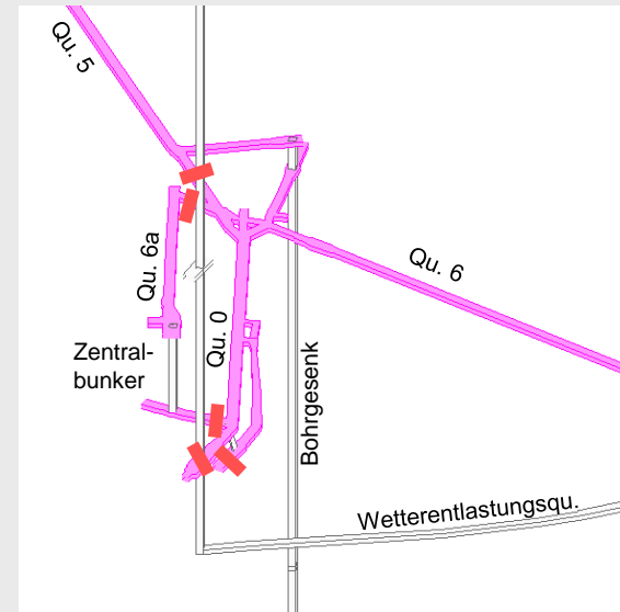
Holzfänger 4. Sohle Oeynhaus 3 (Perspektive)
